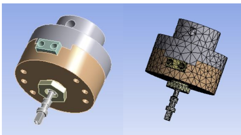
(a) Modello per l'analisi a trazione. (b) Mesh creata per l'analisi a trazione.
