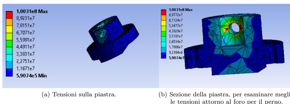
Figura 5.6.: Tensioni sulla piastra superiore del lato dell'afferraggio su cui sono applicati i carichi.
