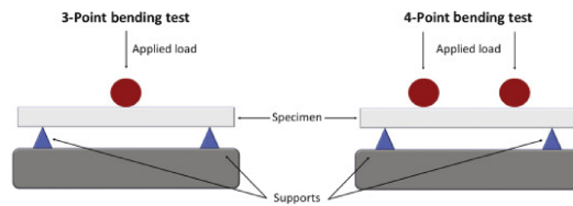
Figura 1.24.: Flessione a 3 e 4 punti.
