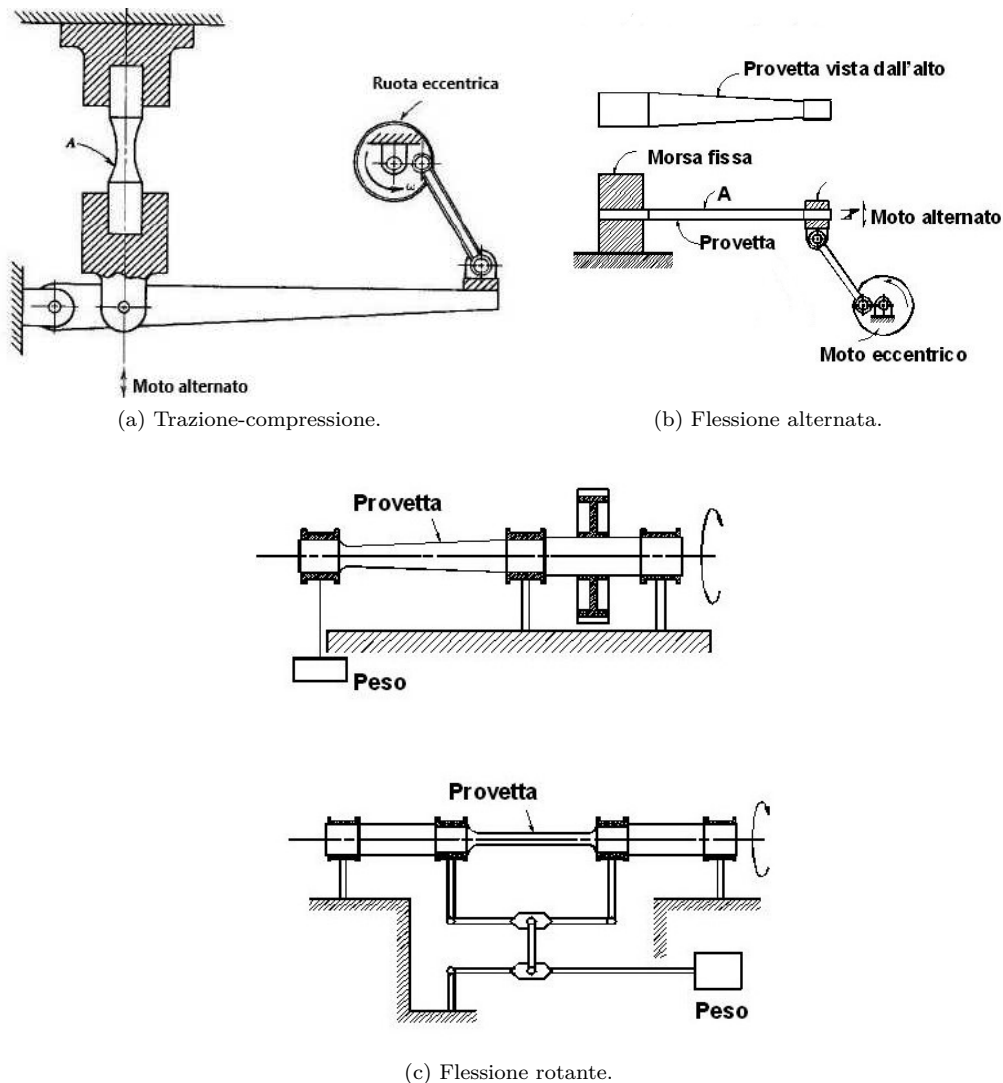
Figura 1.16.: Schema di macchine per prove di fatica.
