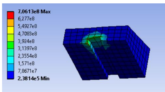
(a) Tensioni nel cuneo.
