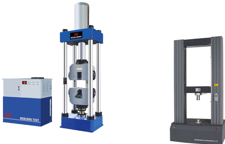
(a) Macchina universale servoidraulica.
