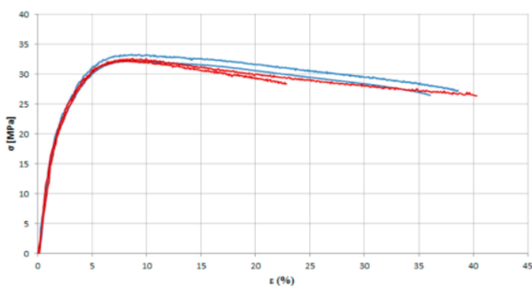
Figura 24 Confronto curve tensione deformazione ottenute dal sistema di sperimentazione biassiale con test distinti tra asse orizzontale e asse verticale.
