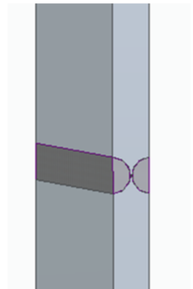
Figura 30. Passaggio dall'accoppiamento di lamiere non saldato a quello in cui si realizza il fissaggio con saldatura "a doppio U"
