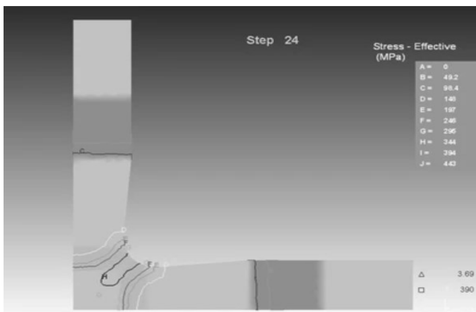
Figura 16. Secondo step di un generico processo di ottimizzazione della geometria del provino
