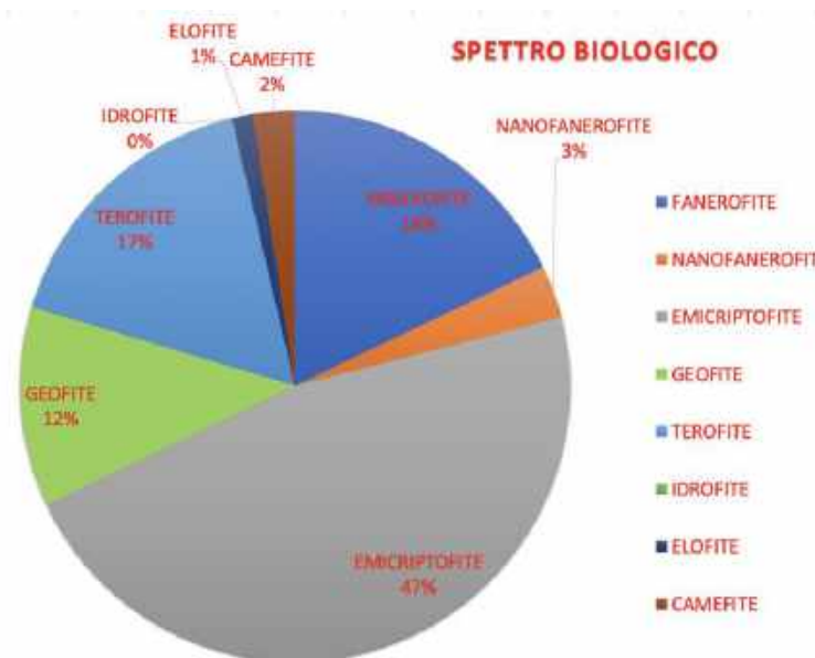
Fig. 38 – Spettro biologico delle specie rilevate attraverso l'analisi floristica.
