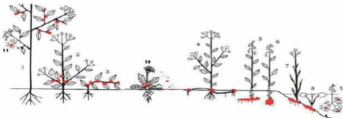
Fig. 8 – Forme biologiche. In rosso la posizione delle gemme che sopravvivono durante la stagione avversa. 1: Fanerofite. 2-3: camefite; 4: Emicriptofite; 5: geofite rizomatose; 6: geofite bulbose; 7: Elofite; 8: Idrofite radicante; 9: Idrofite natante; 10: Terofite rosulate. 11: Fanerofite epifitiche. [Fonte: www.actaplantarum.org ; Modificato da Giuliano Salvai - Febbraio 20, 2010]
