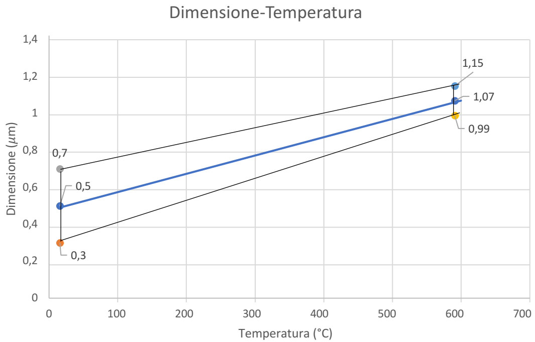
Figura 14 - Variazione della dimensione con l'incremento della temperatura
