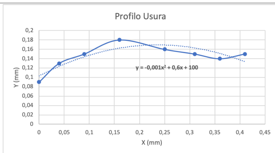
Profilo Usura a T. ambiente (100')
