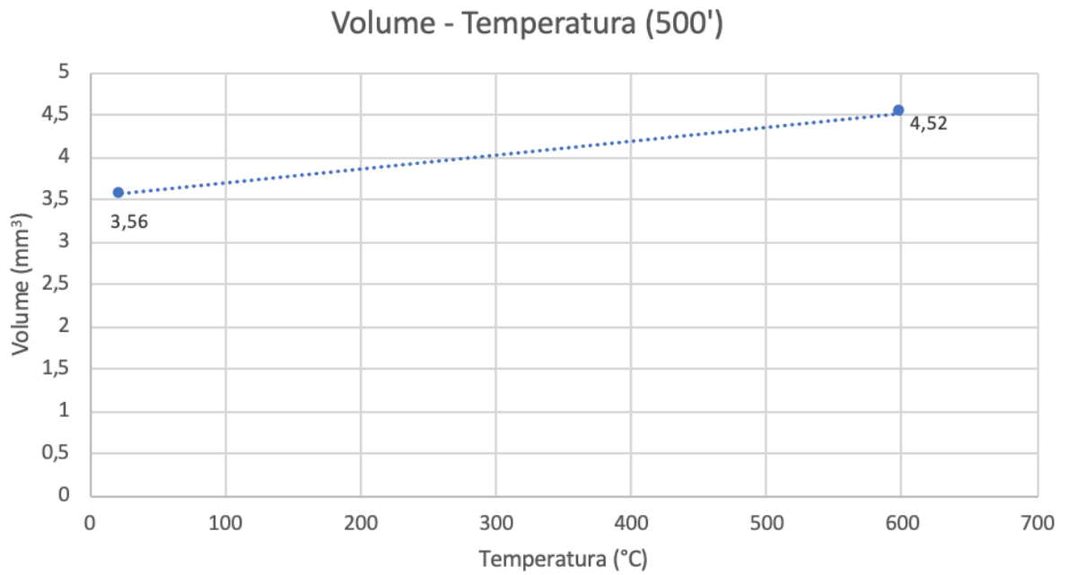
Figura 17 - Variazione volume con l'incremento della temperatura dopo 500 minuti di lavorazione
