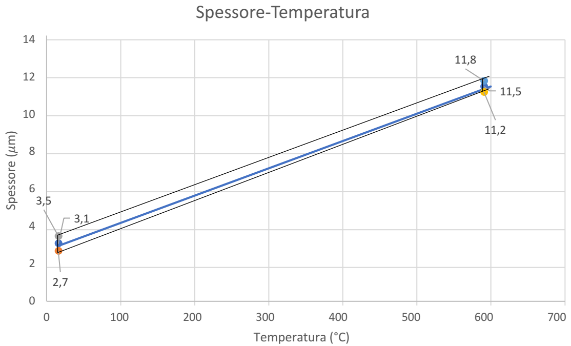
Figura 15 - Variazione dello spessore con l'incremento della temperatura
