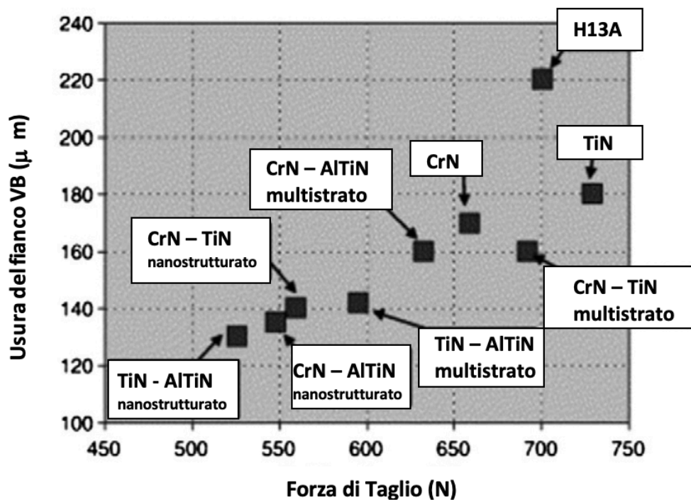
Figura 7 – Usura del fianco (in \mu m) contro la forza di taglio (in N) durante la tornitura di Inconel 718 a 40 m/min con utensili in metallo duro rivestiti con multistrato e nanostrutturati PVD (10).
