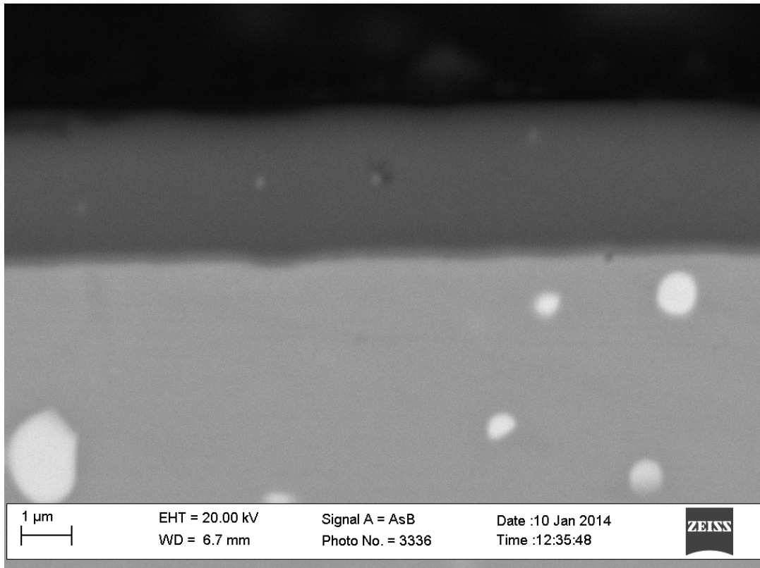
Figura 12 - Micrografia SEM di un acciaio HSS601 con rivestimento multistrato AlTiCrN a temperatura ambiente
