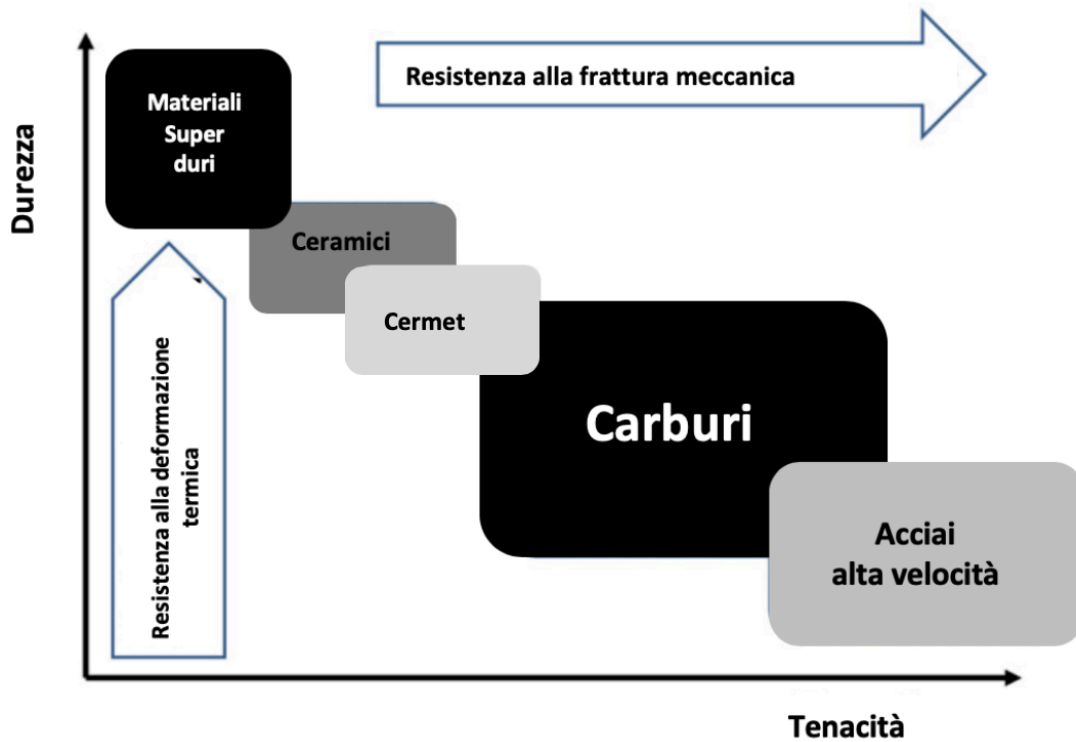
Figura 5 – Materiali usati per la fabbricazione di utensili da taglio e le relative proprietà di durezza/tenacità (7)
